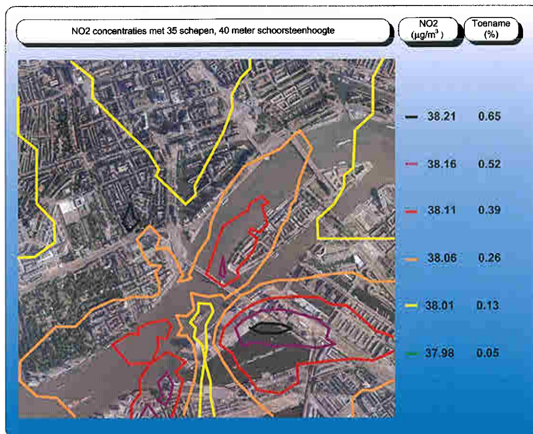
Figuur 5.2: NO 2 concentraties met 35 schepen, 40 m schoorsteenhoogte 31
