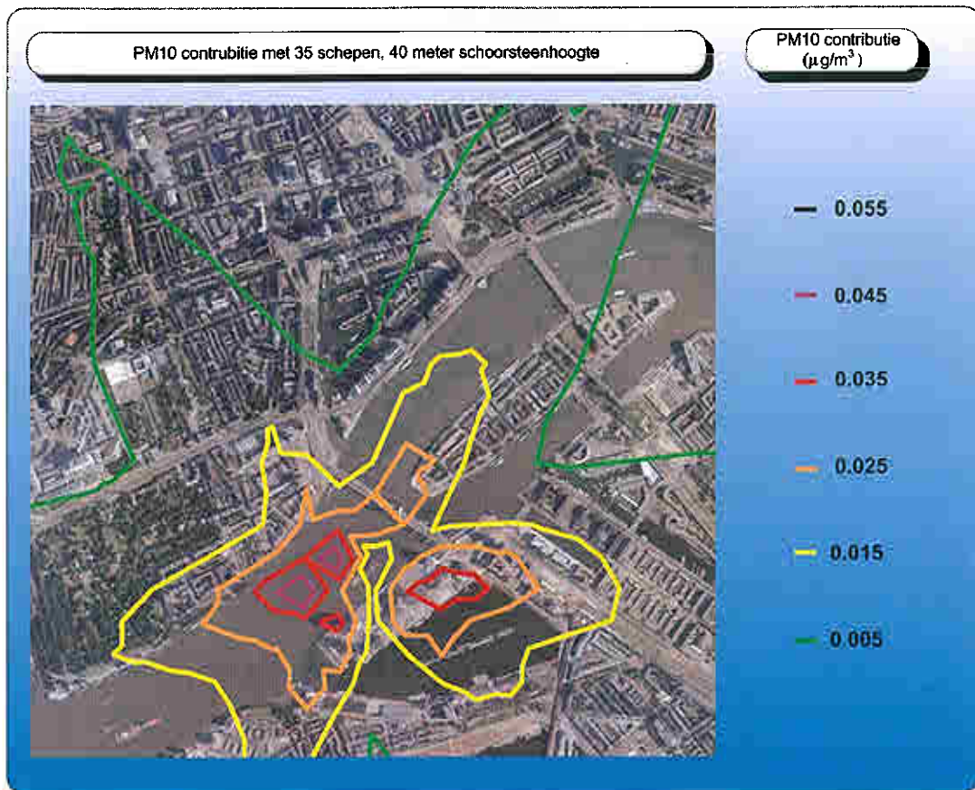
Figuur 5.3 PM 10 concentraties met 35 schepen, 40 m schoorsteenhoogte 32
